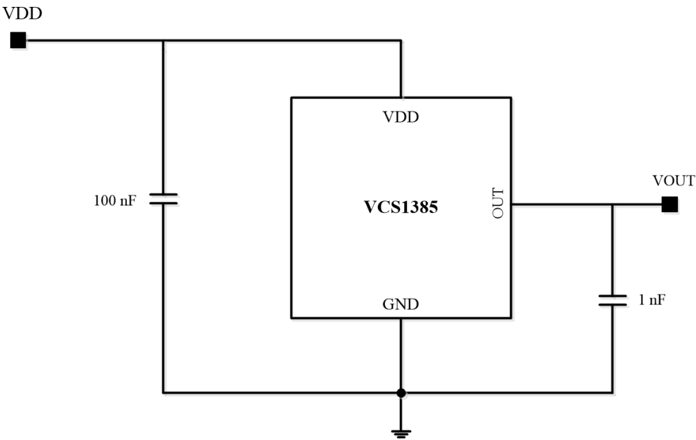
图 6 典型应用电路图
