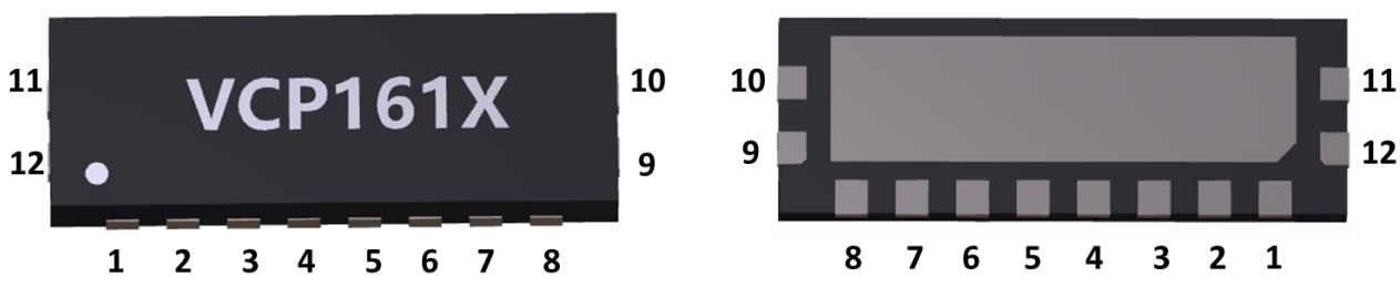
图 3 封装管脚示意图
